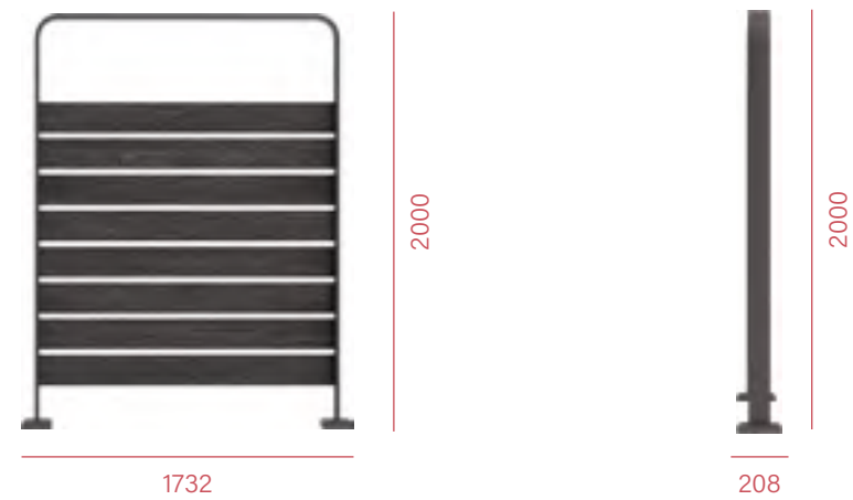
NOMAD DIVIDER - 1732 x 2000
